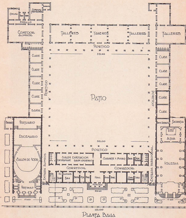
Proyecto de la primera fundación salesiana en Santo Domingo, iniciada por el P. Pittini en 1934 e inaugurada la parte central en 1935. Posteriormente los talleres a la izquierda y la iglesia a la derecha.
