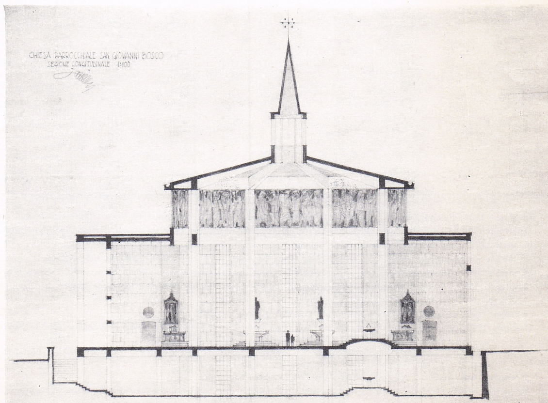
Sezione longitudinale della Chiesa Parrocchiale.
