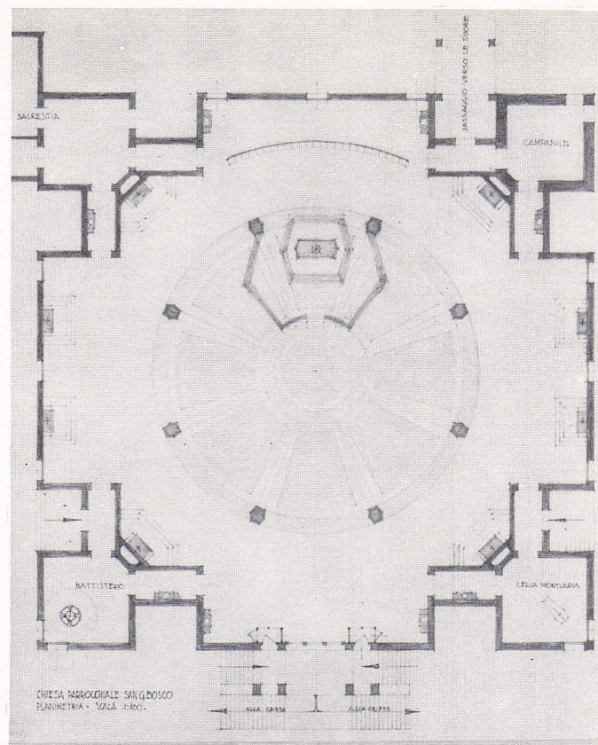
Planimetria della Chiesa Parrocchiale.
