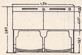
BANCO DI SCUOLA A DUE POSTI
